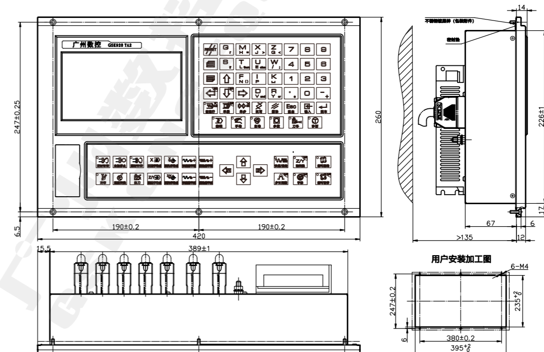
GSK 928TA2外形安装尺寸
